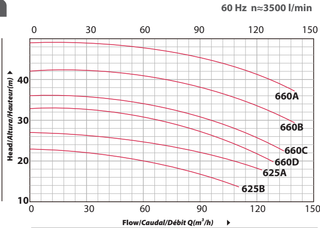
PERFORMANCE CURVE/CURVA DE RENDIMIENTO/COURBE DE PERFORMANCE
